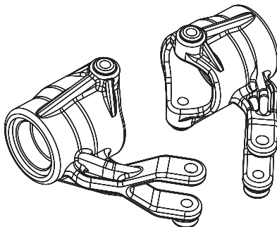
50 040 5261 Lenkhebel l/r vorne Kunststoff Front steering arm l/r plastic
