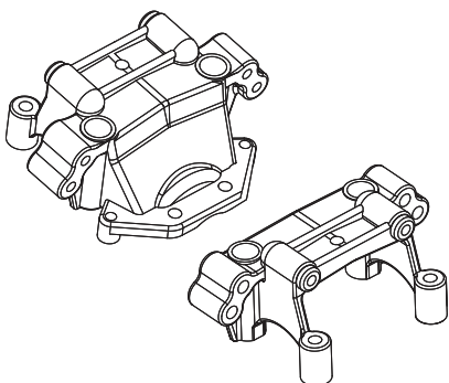
50 040 5258 Querlenkerhalter oben v/h Upper suspension arm mount f/r
