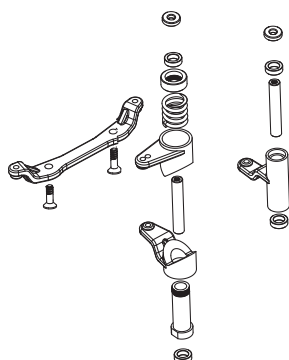
50 040 5272 Lenkservogestängeset Steering servo horn and linkage
