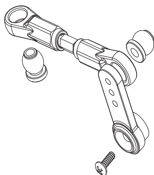
50 040 5273 Radträger hinten L/R Hub rear carrier l/r
