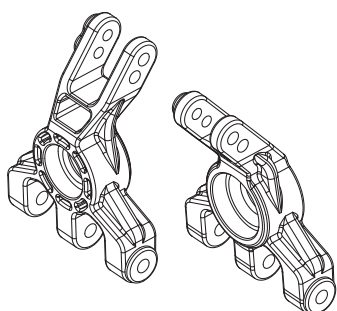
50 040 5273 Radträger hinten L/R Hub rear carrier l/r
